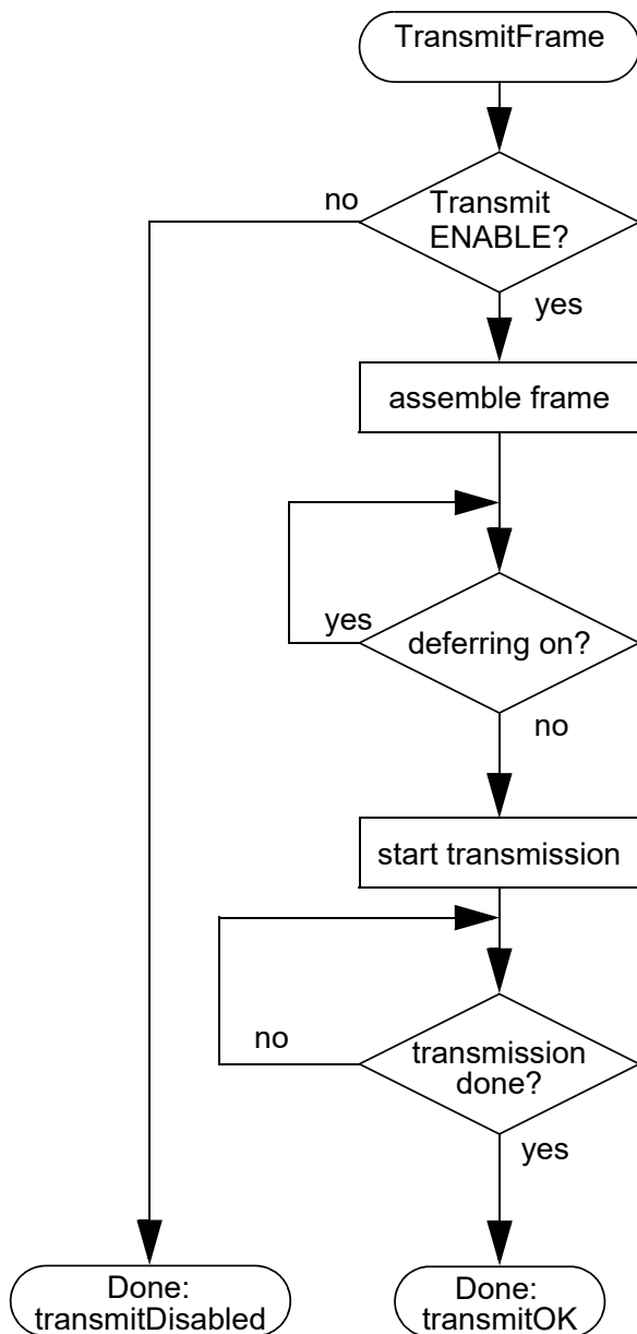
a) TransmitFrame
